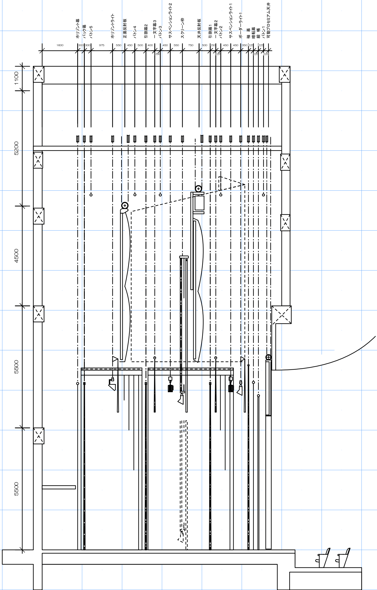
瀬戸蔵 つばきホール 吊物断面配置図 S=1/100
